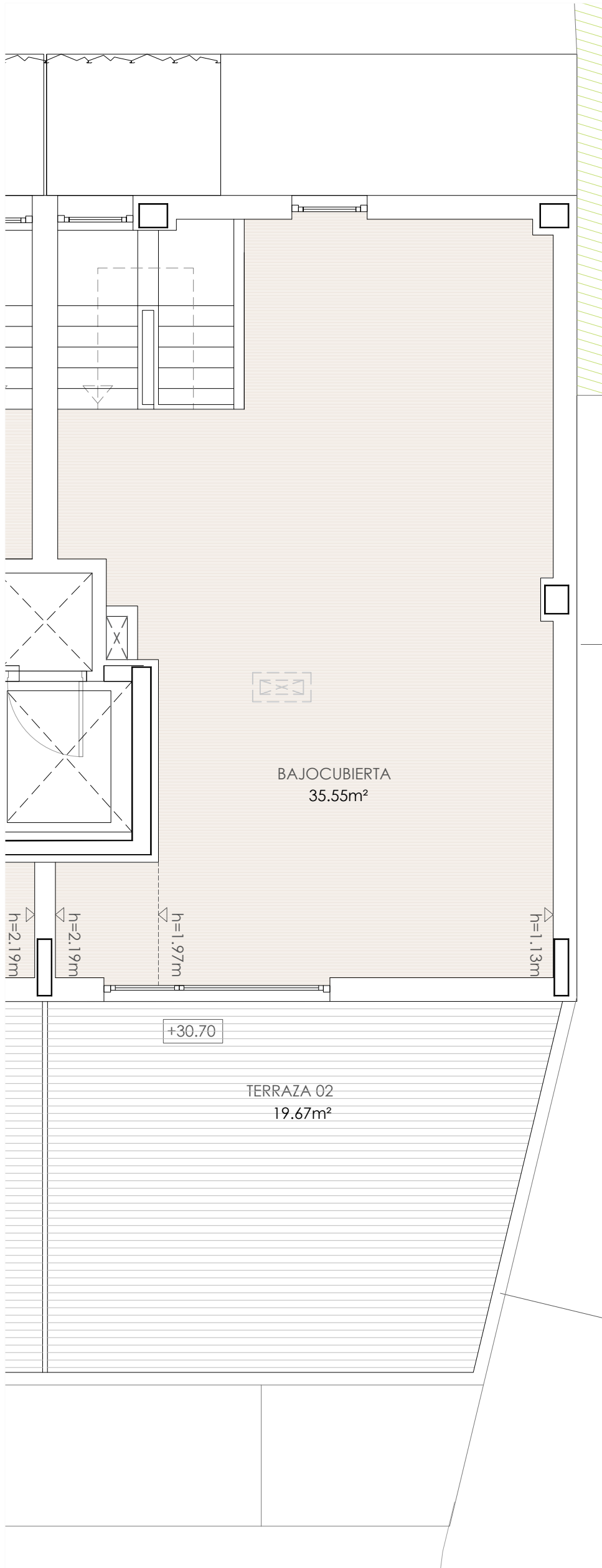
PLANTA BAJOCUBIERTA · VIVIENDA B e: 1/50
