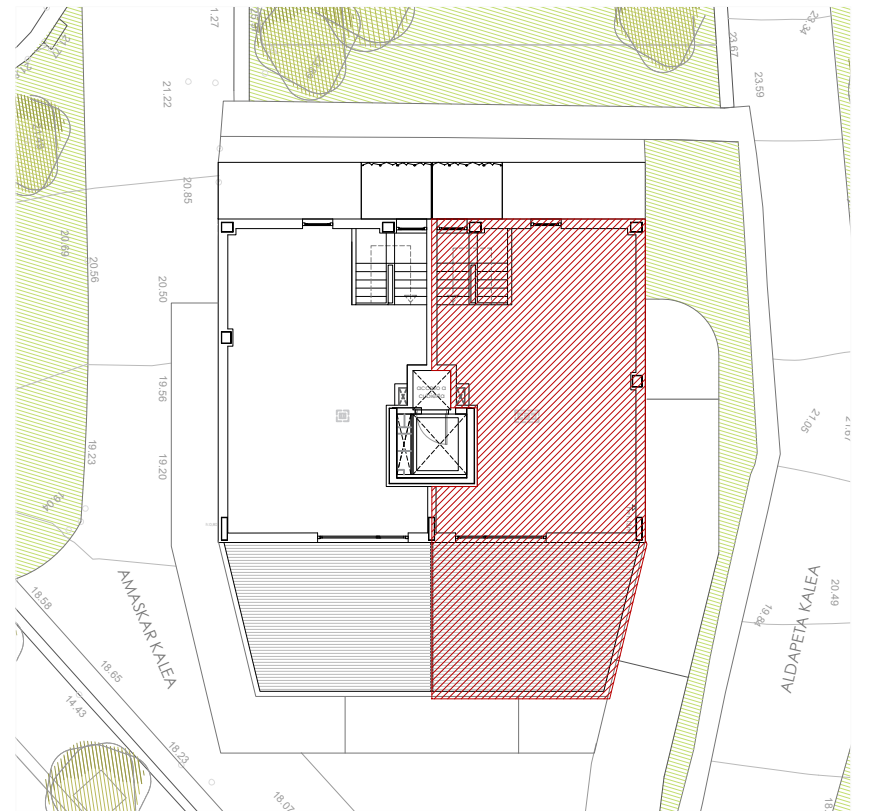
PLANTA BAJOCUBIERTA e: 1/200
